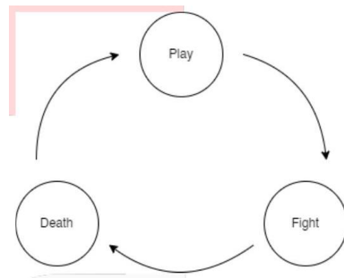
Gambar 1. Perancangan Aplikasi
