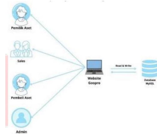
Gambar 1. Arsitektur Aplikasi
