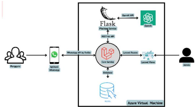
Gambar 1. Arsitektur Aplikasi
