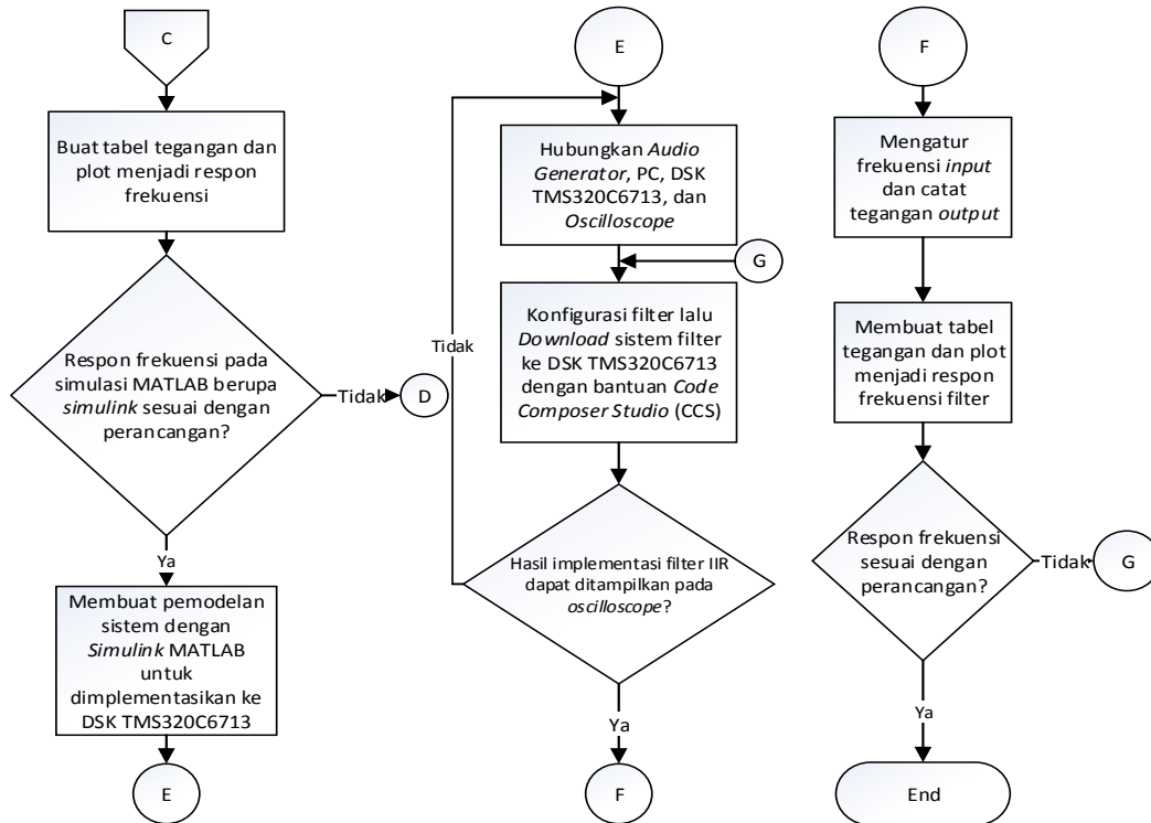
Gambar 4. Diagram Alir Implementasi Filter IIR (lanjutan)
