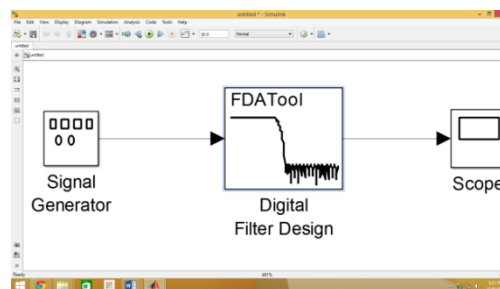
Gambar 1. Blok rangkaian simulasi filter IIR menggunakan Simulink
