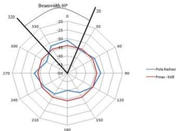
Gambar 10. Beamwidth Vertikal
