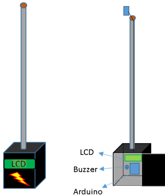
Gambar 2. Gambaran Alat
