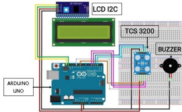
Gambar 4. Skematik Rangkaian
