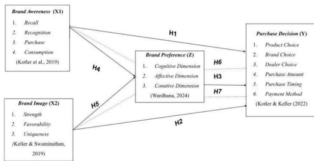
Gambar 3. Kerangka Pemikiran
