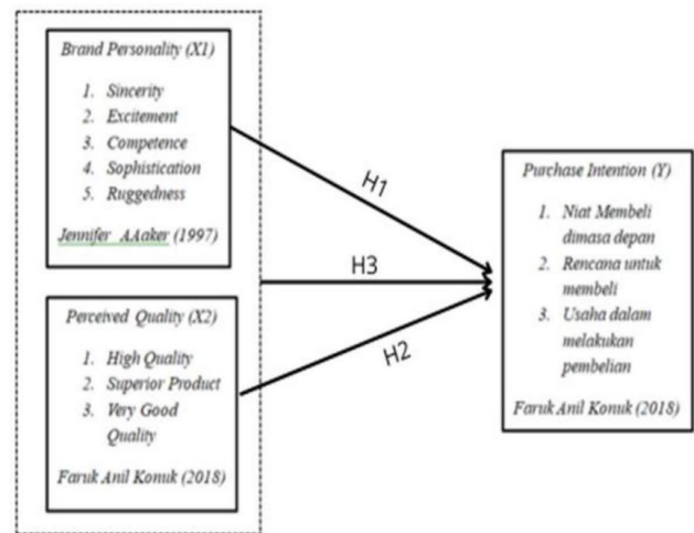
Gambar 1. Kerangka Pemikiran
