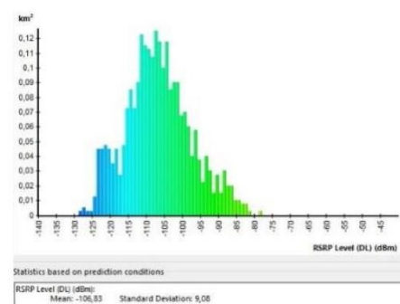
Gambar 13. RSRP Optimasi
