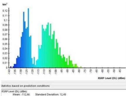
Gambar 12. RSRP Optimasi
