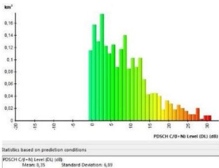
Gambar 11. SINR Optimasi
