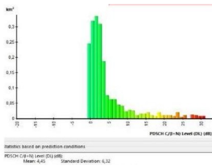
Gambar 10. SINR Awal
