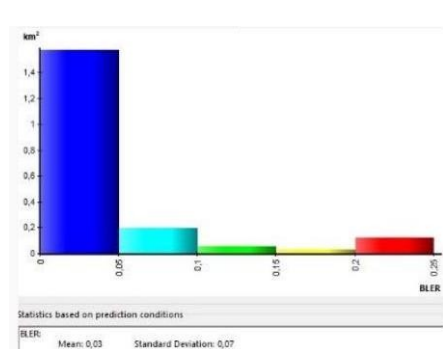
Gambar 15. RSRQ Optimasi
