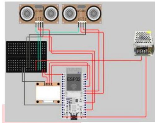
Gambar 3. Wiring Sistem parkir pintar
