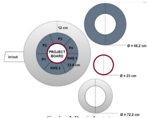
Gambar 2. Desain Layout
