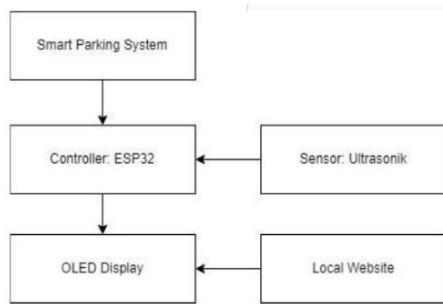
Gambar 1. Diagram Blok Sistem Parkir Pintar
