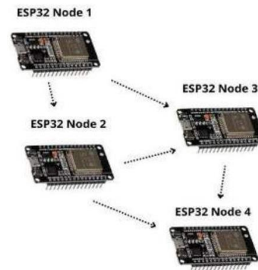
Gambar 11 Topologi Semi-Mesh Menggunakan ESP-NOW
