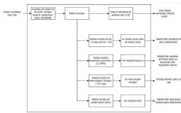
Gambar 8. Diagram blok sistem
