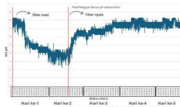
Gambar 13. Hasil Grafik pH terhadap waktu ketika pompa dinyalakan
