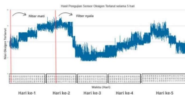
Gambar 15. Hasil Grafik Oksigen Terlarut terhadap waktu ketika pompa dinyalakan
