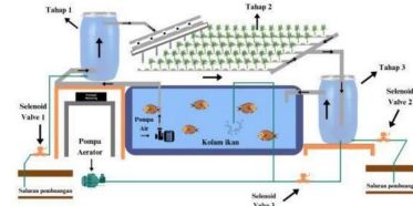
Gambar 1. Sistem akuaponik NFT
