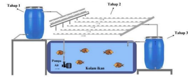
Gambar 3. Penempatan media filter berdasarkan fungsinya
