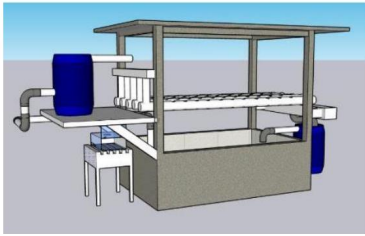
Gambar 9. Desain 3d Kolam Akuaponik
