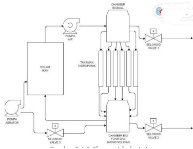
Gambar 2. Skema sirkulasi air
