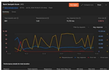
Gambar 9. Pengujian Beban Pada Postman.
