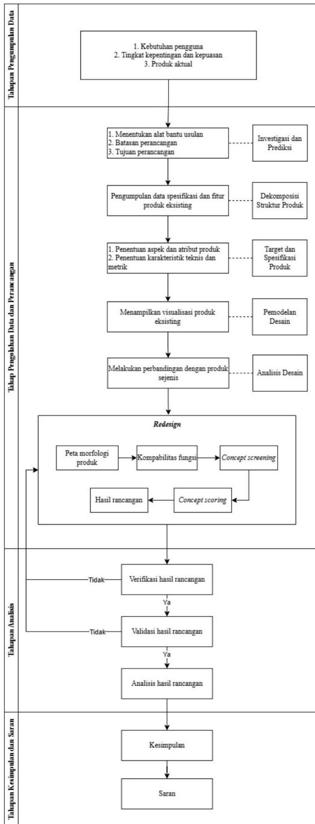
Gambar 3. Sistematika Perancangan
