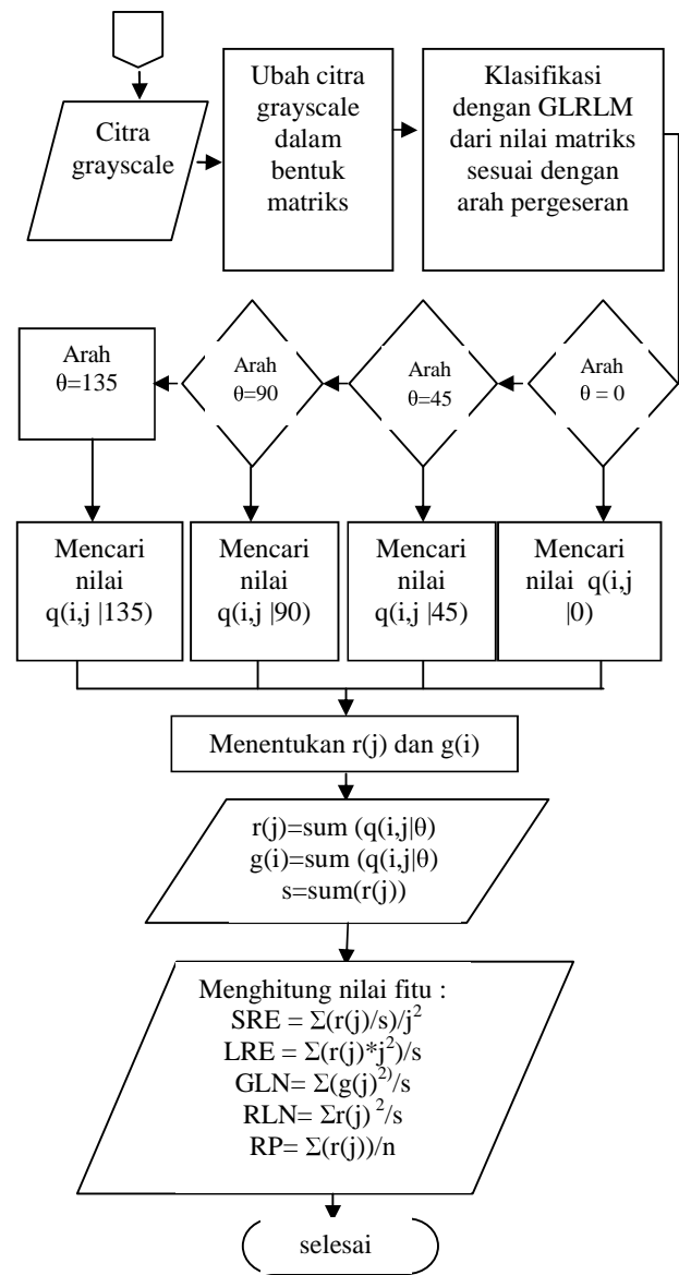
Gambar 5. Bagan Alir Tahap Klasifikasi GLRLM
