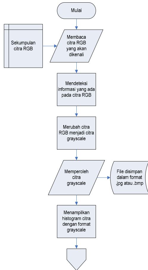
Gambar 4. Bagan Alir Tahap Konversi Citra
