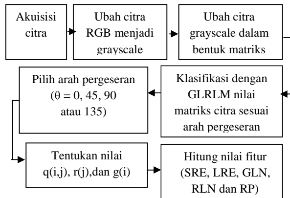
Gambar 3. Gambaran Umum Klasifikasi Tekstur Parket Kayu dengan GRLM
